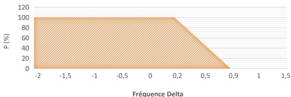
Exemple de fonction de l'onduleur PV illustrant la puissance en fonction de la fréquence delta
